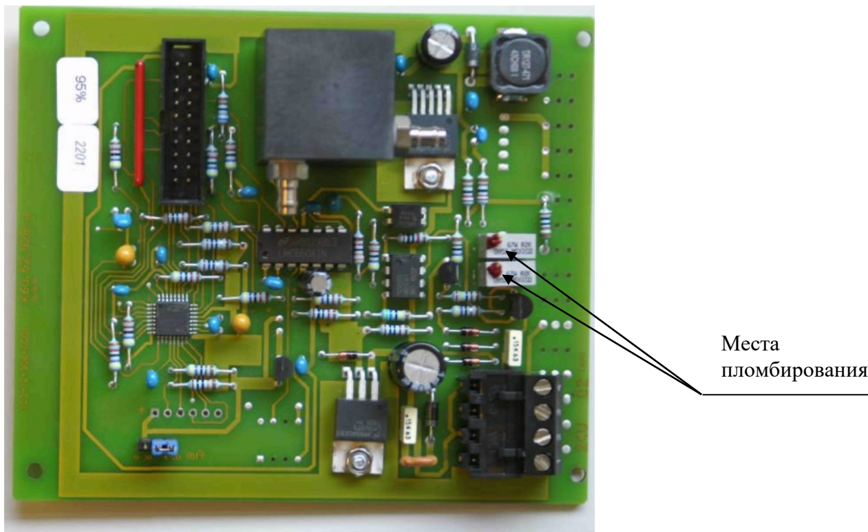
Рисунок 1 Общий вид модуля газового анализа кислородного FCX-MCxx-CN
