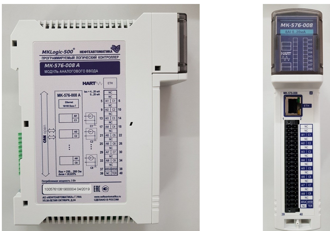
Рисунок 8 – Внешний вид модуля аналогового ввода МК-576-008 А.
