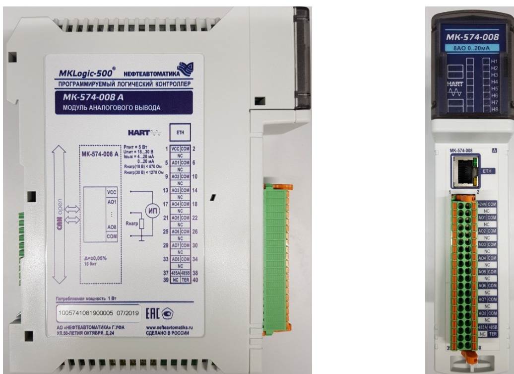
Рисунок 9 – Внешний вид модуля аналогового вывода МК-574-008 А.
