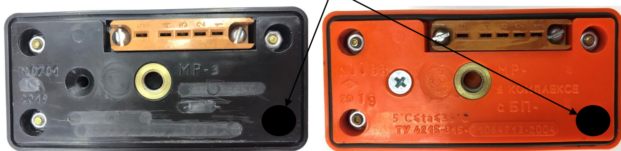
а) б) а) – Метанометры МГМ-1М б) – Метанометры МГМ-1.1М и МГМ-1Р
