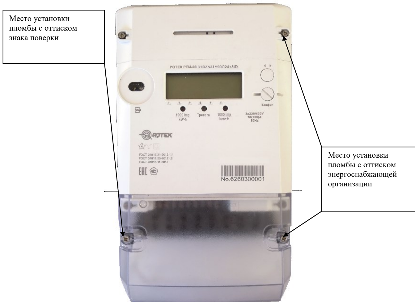
Рисунок 1 – Общий вид счетчиков и схема пломбировки от несанкционированного доступа
