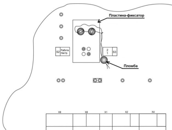
Р и с у н о к 4 – Схема пломбировки от несанкционированного доступа электронно-вычислительного устройства (счетчика) производства ООО "Топаз-сервис", г. Волгодонск
