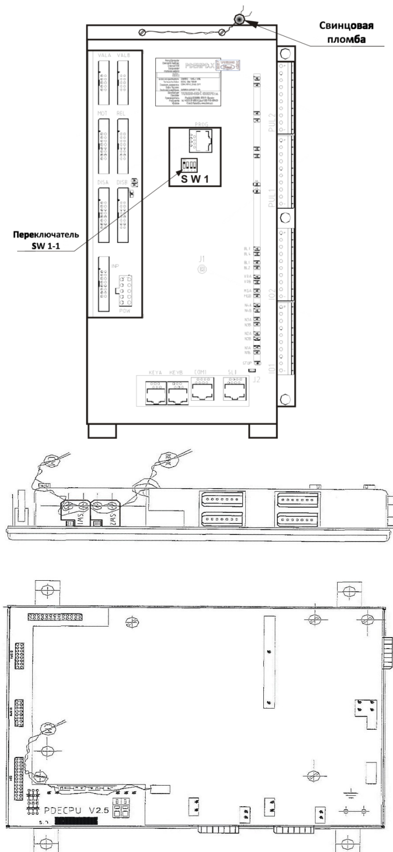
Р и с у н о к 3 – Схема пломбировки от несанкционированного доступа электронно-вычислительного устройства (счетчика) производства TATSUNO EUROPE a.s. (Чешская республика)
