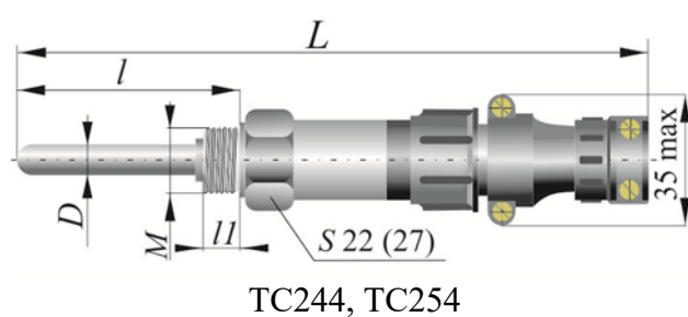
Рисунок 5 – Общий вид термопреобразователей сопротивления TC004
