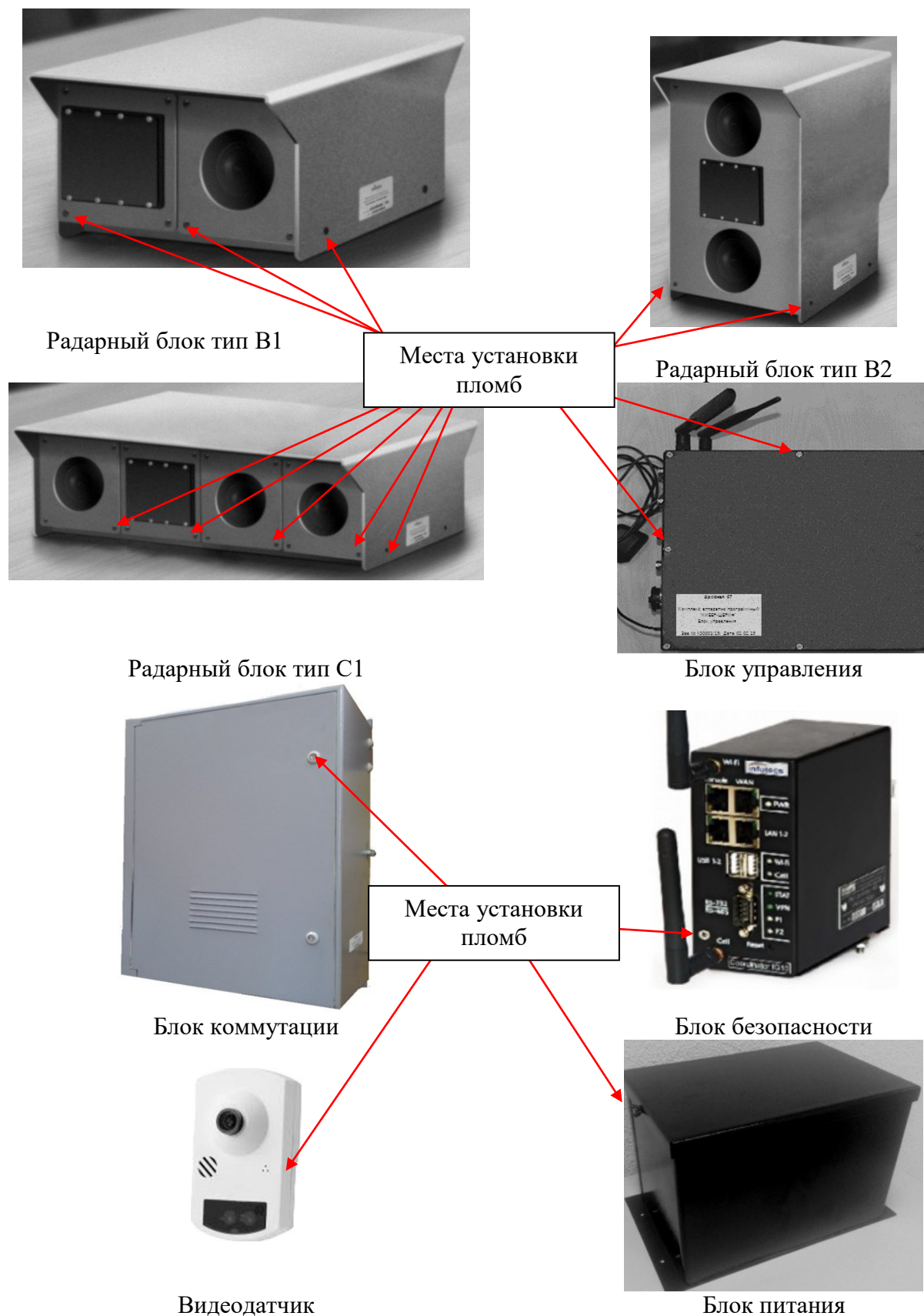
Рисунок 1 – Общий вид составных частей комплекса и места установки пломб
