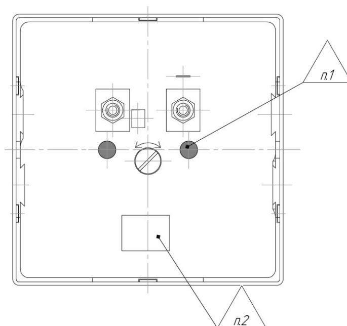
Рисунок 2 – Место ограничения доступа к местам настройки (регулировки) и место нанесения знака поверки миллиамперметров, амперметров и вольтметров М42408, вольтметров Ц42408
