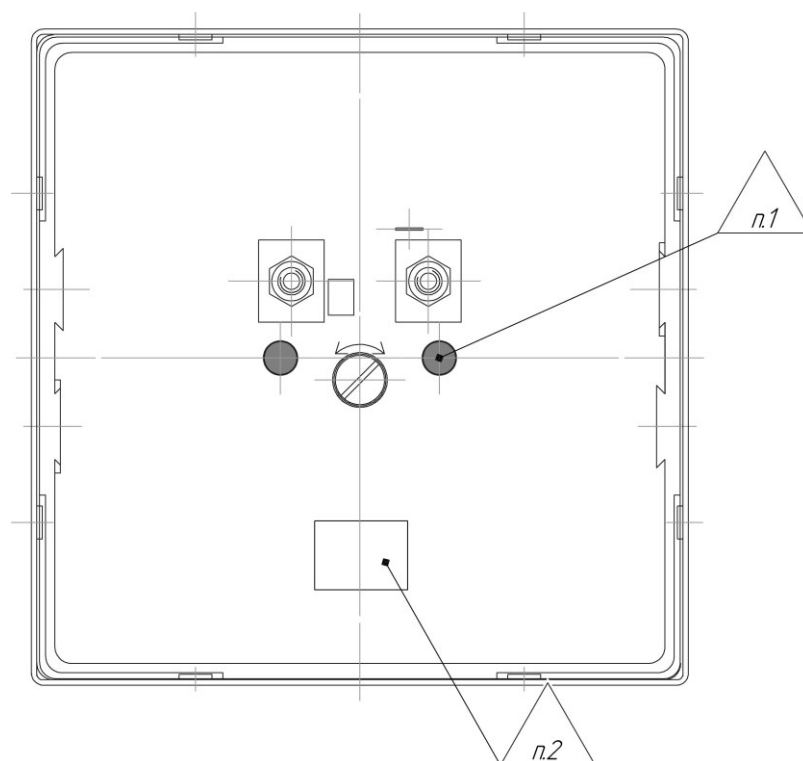
п. 1 – место ограничения доступа к местам настройки (регулировки) (клеймо ОТК) п. 2 – место нанесения знака поверки
