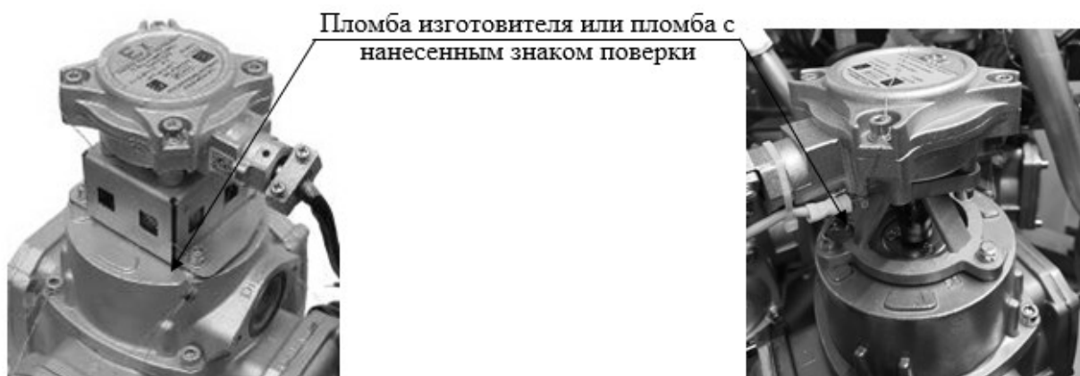
Рисунок 10 – Схемы пломбировки генераторов импульсов
