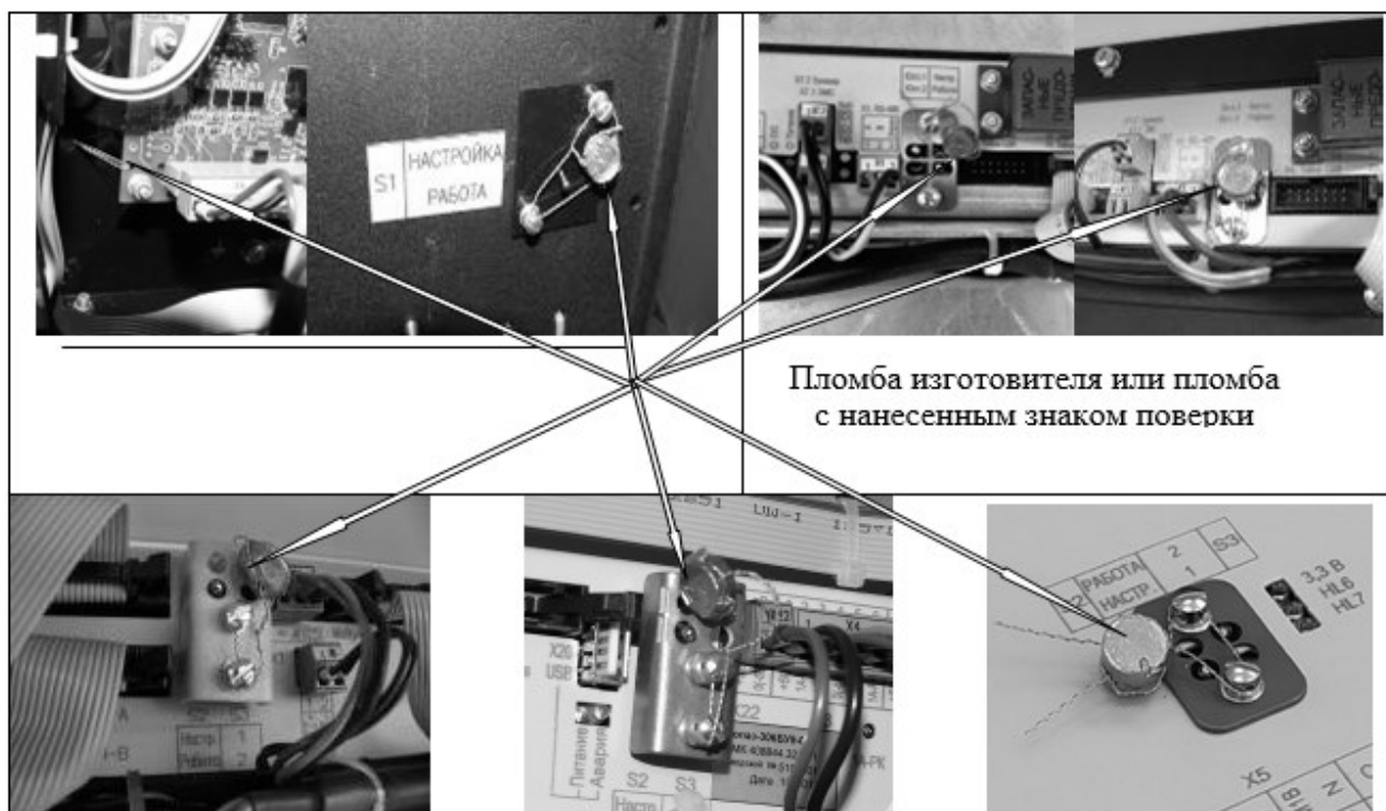
Рисунок 14 – Схемы пломбировки блоков управления «Топаз-306БУ»
