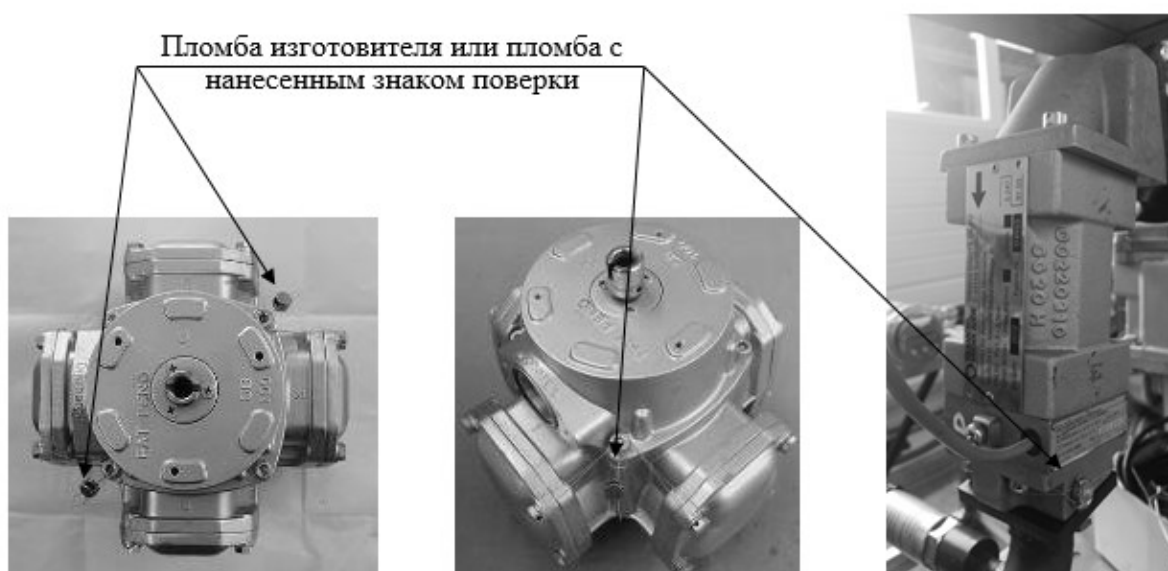
Рисунок 11 – Схема пломбировки измерителей объёма
