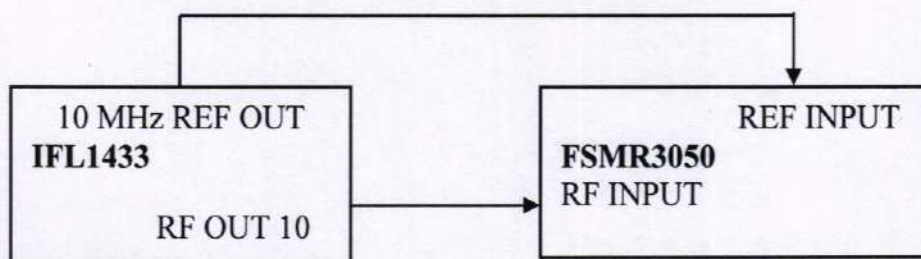
Рисунок 5 – Структурная схема соединения СИ для определения абсолютной погрешности установки коэффициента амплитудной модуляции и абсолютной погрешности установки девиации частоты
