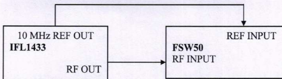
Рисунок 6 – Структурная схема соединения СИ для определения коэффициента подавления сигнала несущей в паузе между радиоимпульсами
