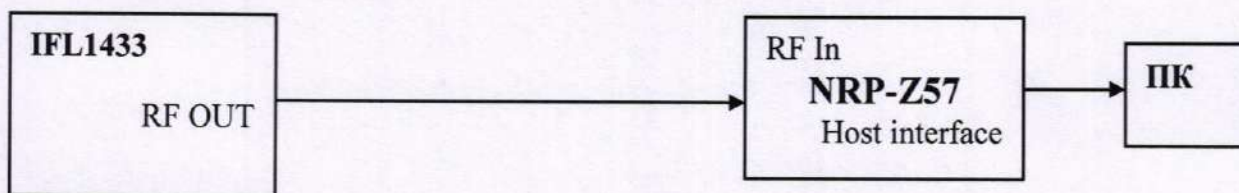
Рисунок 2 – Структурная схема соединения СИ для определения абсолютной погрешности установки уровня мощности выходного сигнала
