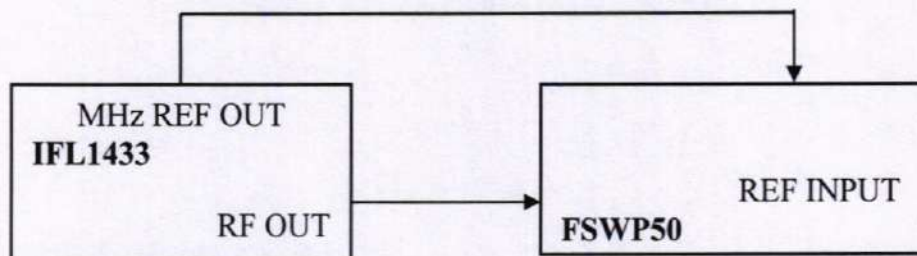
Рисунок 3 – Структурная схема соединения СИ для определения абсолютной погрешности установки уровня мощности выходного сигнала в диапазоне от минимального значения до минус 10 дБ (1 мВт)
