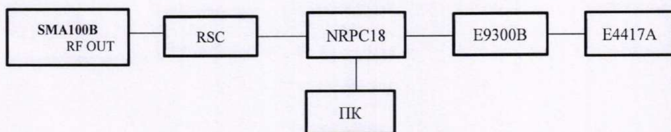
Рисунок 3 – Структурная схема соединения СИ для определения относительной погрешности измерений уровня мощности минус 30 дБ (1 мВт)
