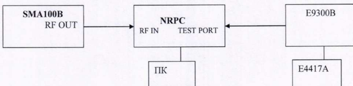
Рисунок 2 – Структурная схема определения относительной погрешности измерений мощности на опорном уровне 1 мВт
