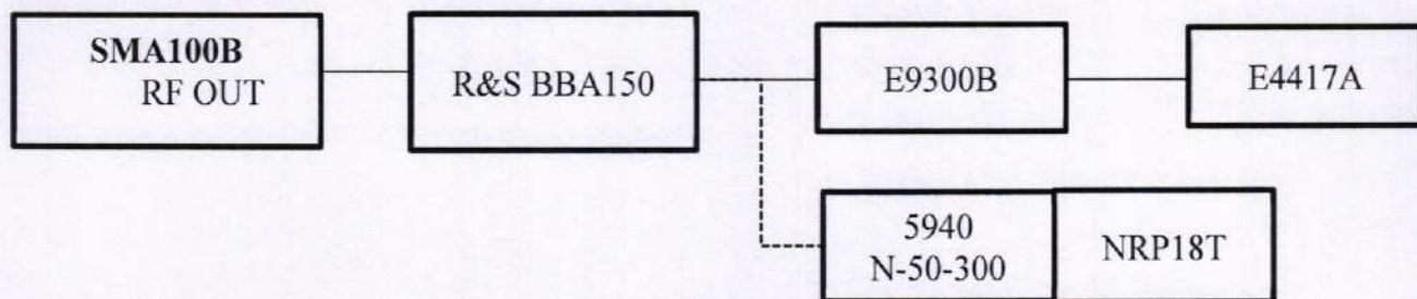
Рисунок 4 – Структурная схема соединения СИ для определения относительной погрешности измерений уровня мощности 44 дБ (1 мВт)
