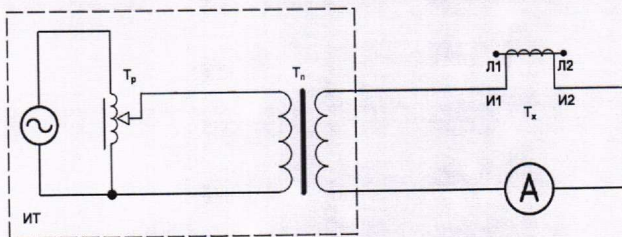
Рисунок 2 – Схема размагничивания трансформатора вторым способом
