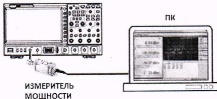
Рисунок 4 – Схема подключения оборудования при определении неравномерности амплитудно-частотной характеристики генератора
