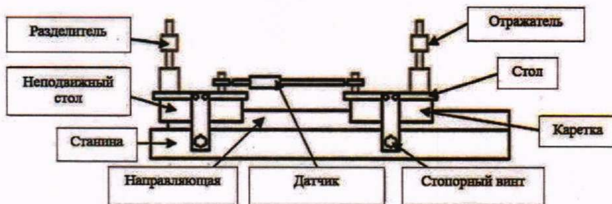
Рисунок 1 – Внешний вид устройства для линейного позиционирования и схема установки датчика
