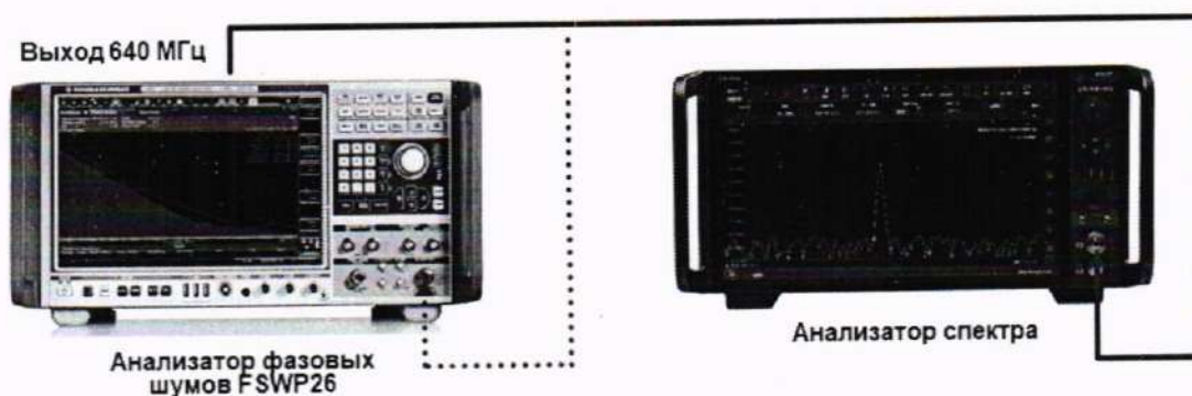
Рисунок 7 - Схема соединения приборов для определения спектральной плотности фазовых шумов
