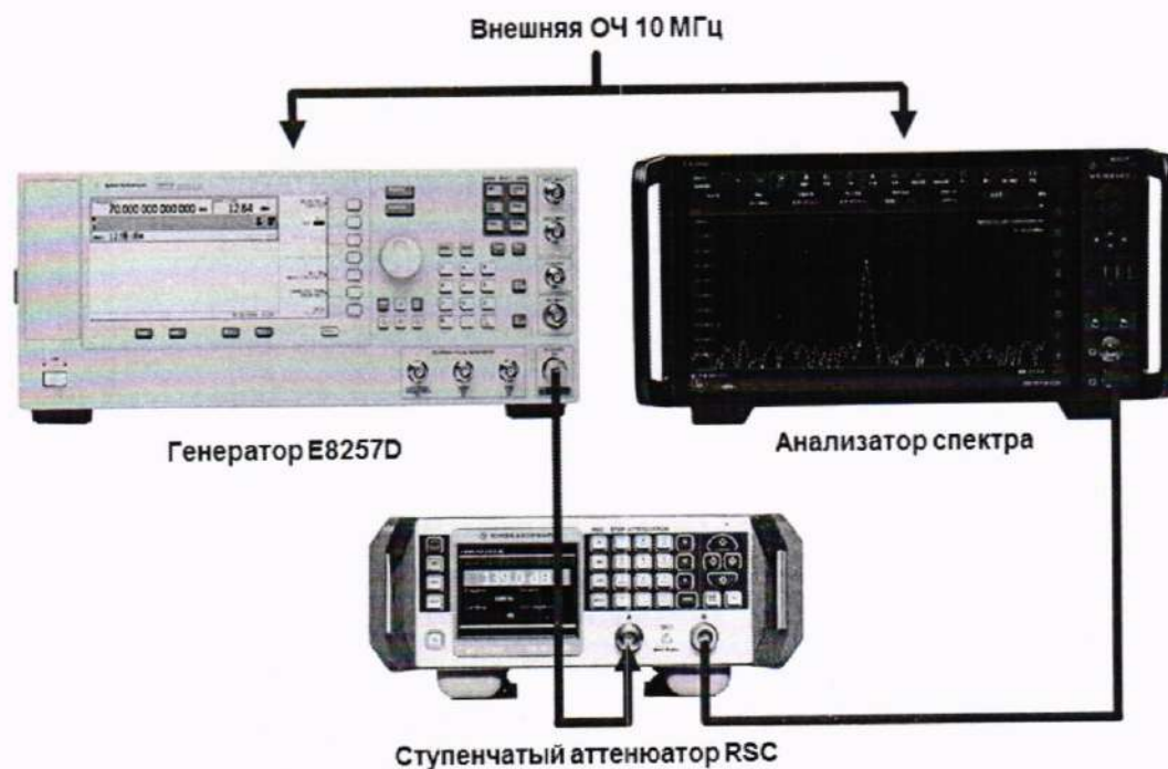
Рисунок 3. Схема соединения для определения абсолютной погрешности установки опорного уровня в диапазоне от минус 60 до минус 10 дБм.
