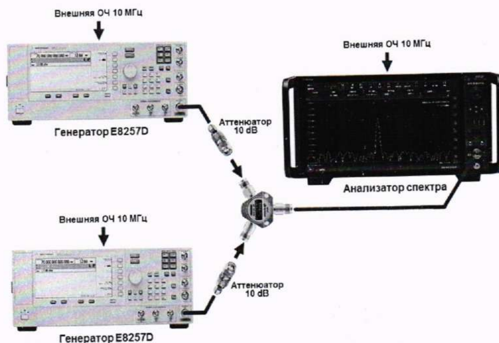
Рисунок 9. Схема соединения приборов для определения уровня интермодуляционных искажений 3-го порядка
