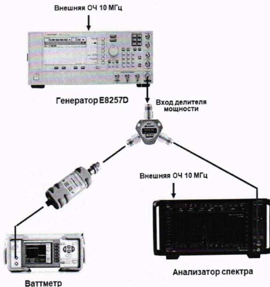
Рисунок 2. Схема соединения для определения абсолютной погрешности измерения опорного уровня
