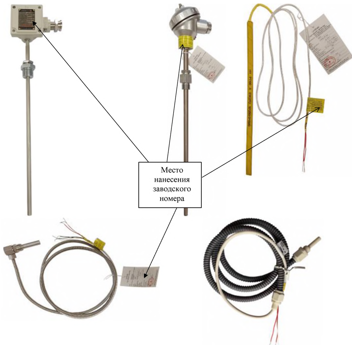
Рисунок 1 – Общий вид термопреобразователей сопротивления платиновых WZ с указанием мест нанесения заводского номера
