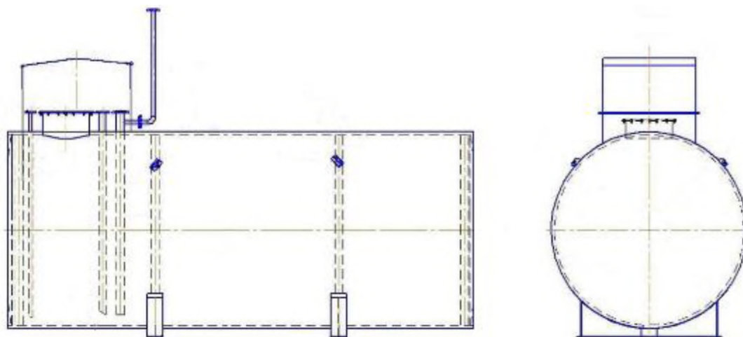
Рисунок 1 – Эскиз общего вида резервуаров РГС-10
