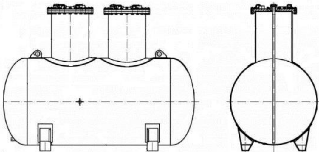
Рисунок 1 – Эскиз общего вида резервуаров РГС-50
