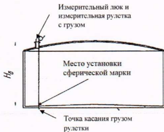
Рисунок А. 1 - Схема измерения базовой высоты резервуара и эталонного расстояния уровнемера
