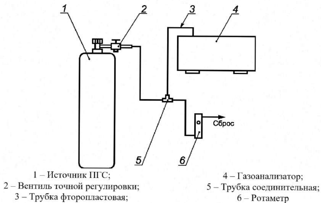
Рисунок В.1 – Рекомендуемая схема подачи ГС на вход газоанализатора
