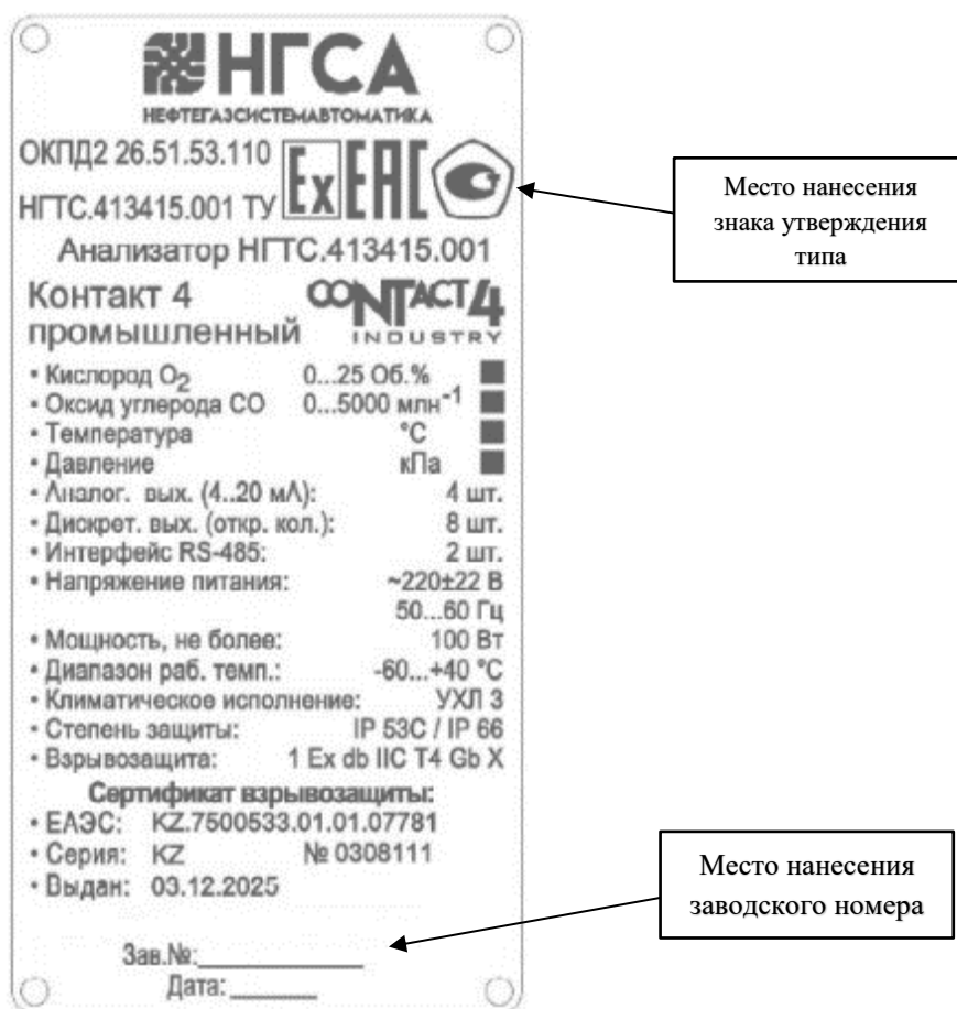
Рисунок 2 – Идентификационная табличка
