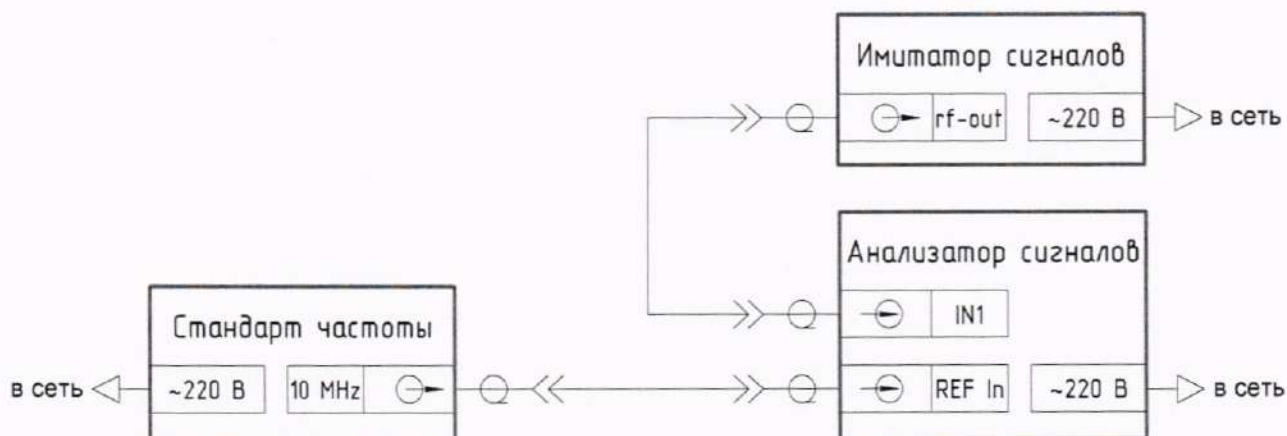
Рисунок 2 — Схема измерений для определения номинальных значений выходных частот
