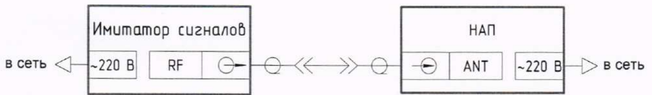
Рисунок 1 — Схема измерений для проведения опробования имитатора сигналов
