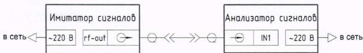
Рисунок 4 — Схема измерений для определения максимального уровня мощности выходного сигнала
