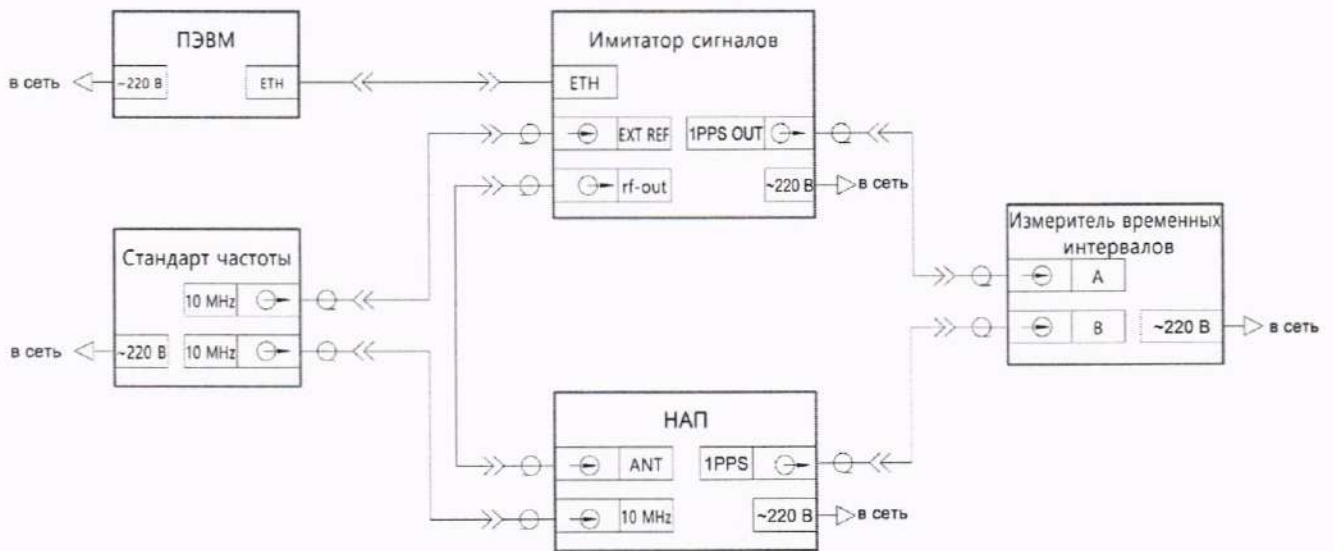
Рисунок 5 — Схема измерений для определения погрешности воспроизведения беззапросной дальности
