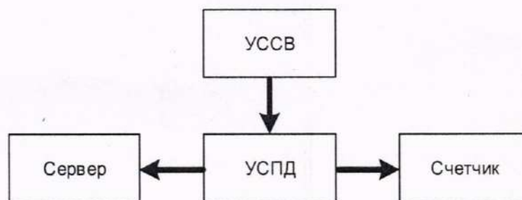
Рис. 2 – Логический канал передачи национальной шкалы времени UTC(SU) от резервного источника точного времени к компонентам СОЕВ
