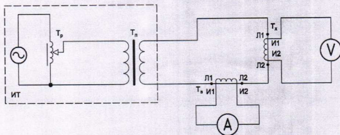
Рисунок 1 – Схема размагничивания трансформатора первым способом
