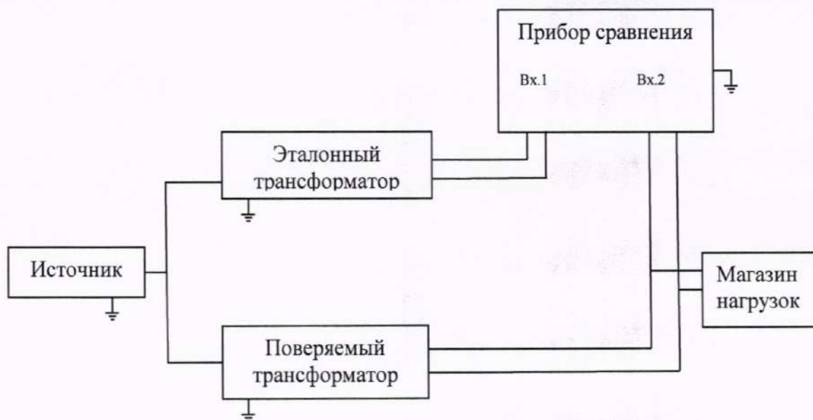
Рисунок 4 – Схема определения токовых погрешностей трансформаторов
