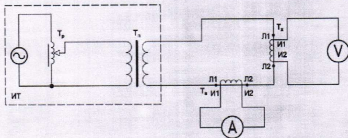
Рисунок 1 – Схема размагничивания трансформатора первым способом
