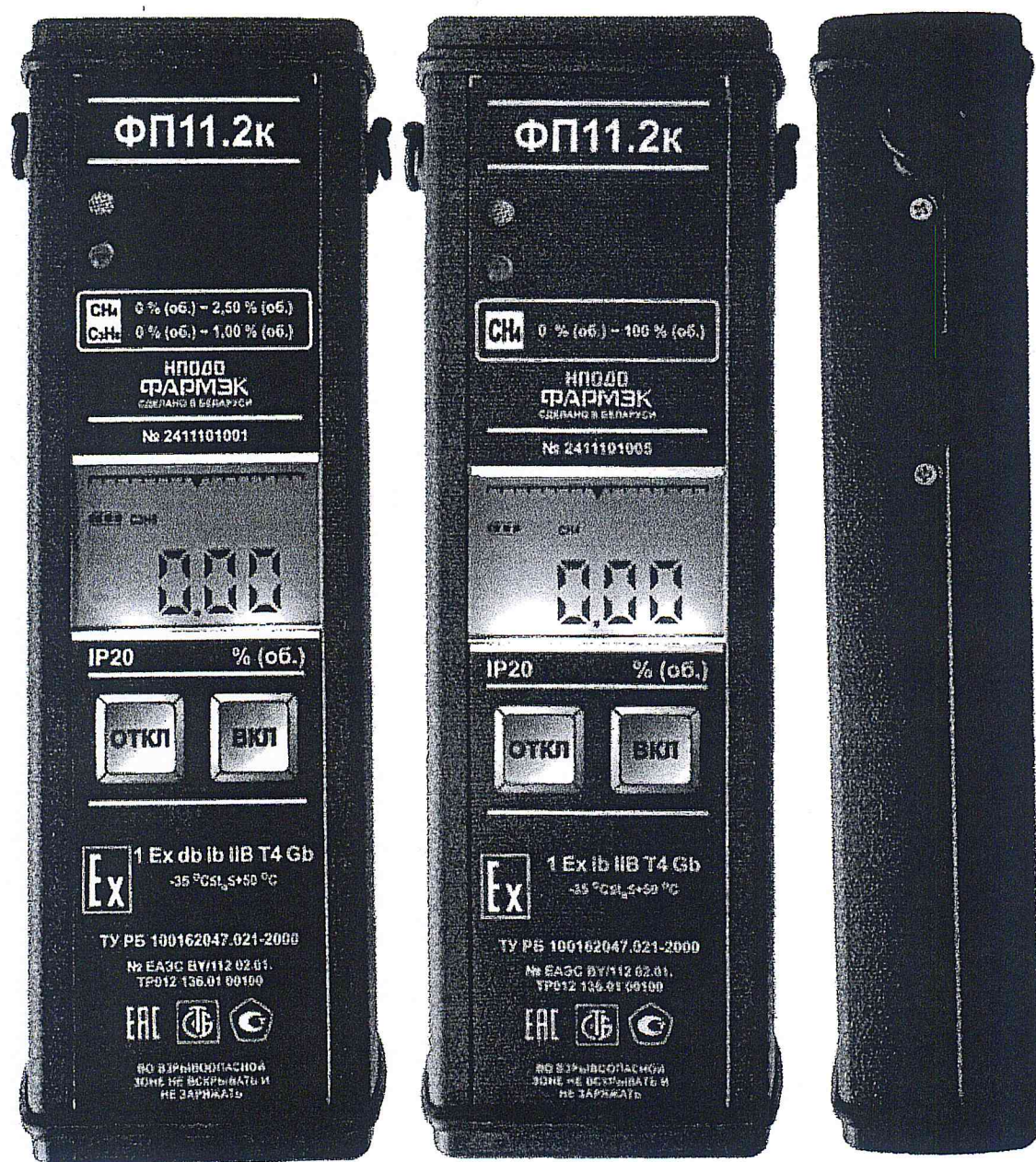
Рисунок 1.1 – Фотографии общего вида и маркировки газоанализаторов ФП11.2к (изображение носит иллюстративный характер)
