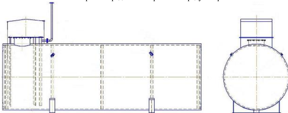
Рисунок 1 – Эскиз общего вида резервуаров РГС-25
