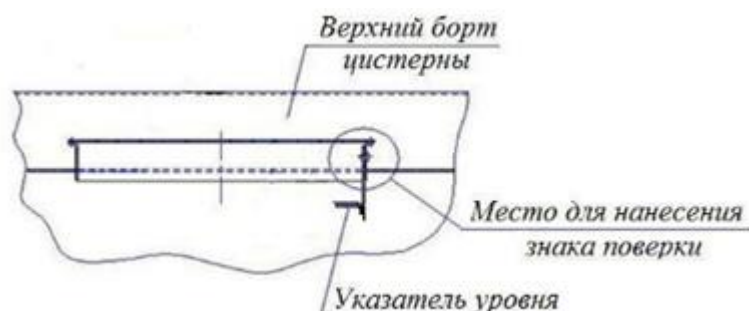
Рисунок 2 – Схема пломбировки от несанкционированного изменения положения указателя уровня налива, обозначение места нанесения знака поверки
