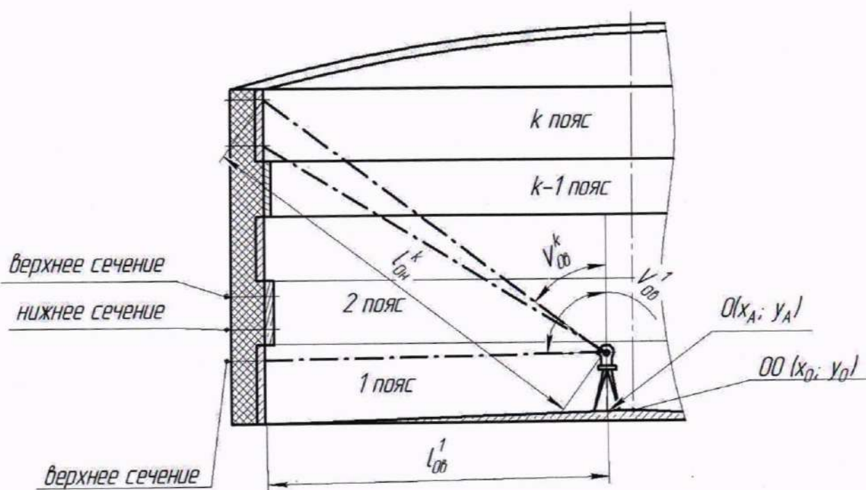
Рисунок А.5 – Схема измерений радиусов поясов резервуара
