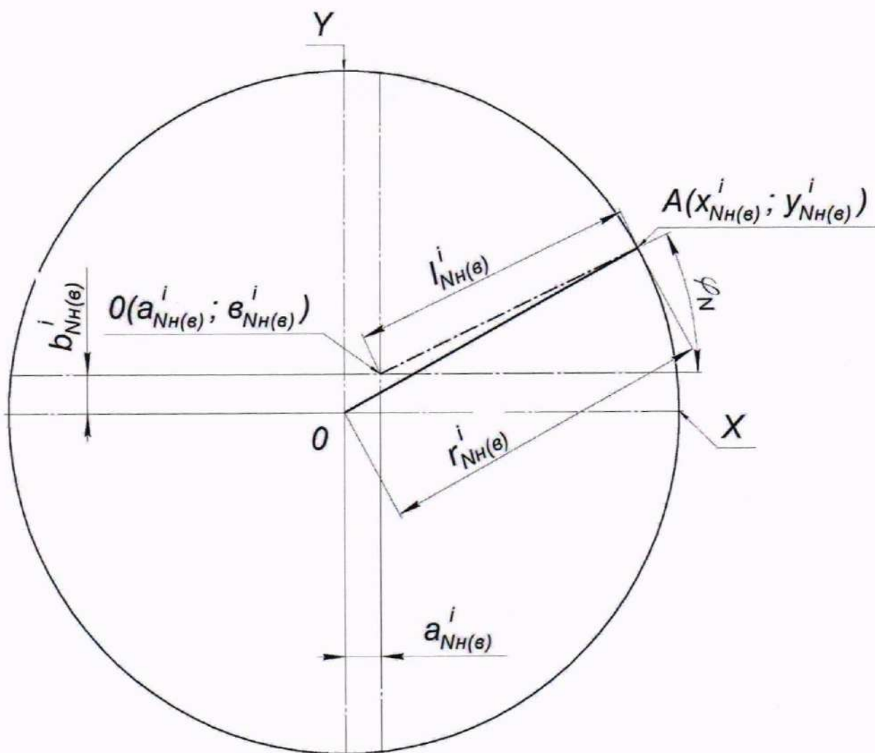
Рисунок Г.1 – Параметры измерений радиуса r_{NH(ε)}^i i -го пояса при j -ом измерении в нижнем (верхнем) сечении
