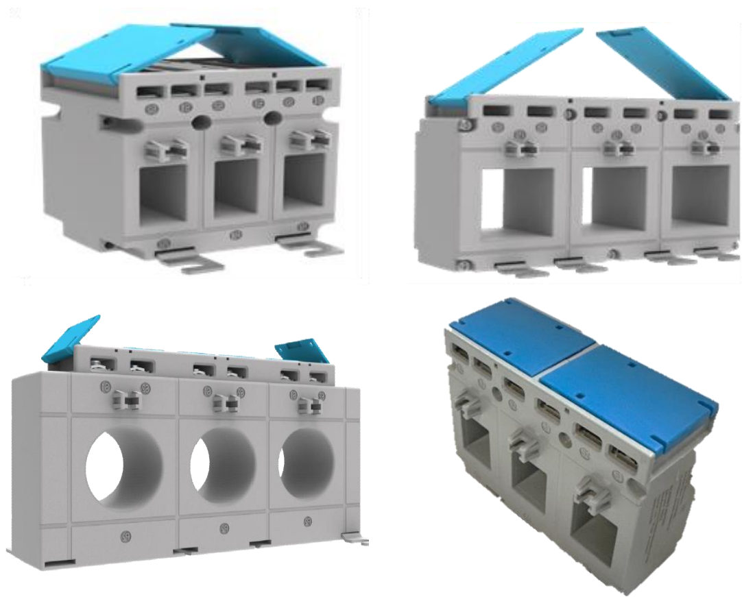
а) серии Ziegler МАК СТ ЗРН
