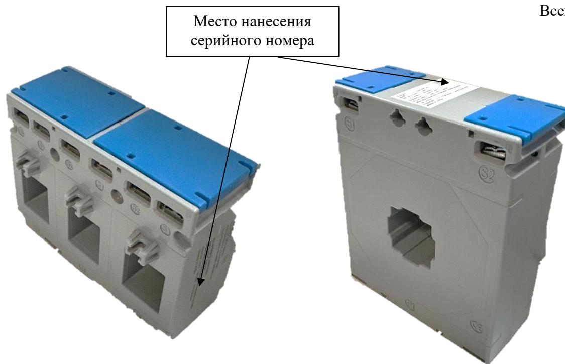
Рисунок 2 – Общий вид трансформаторов тока с указанием места нанесения серийного номера и места нанесения знака поверки
