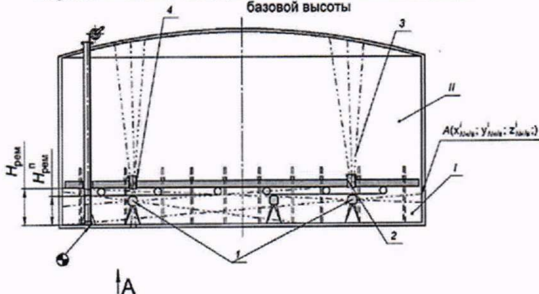
Рисунок А1 – Схема резервуара РВС- 400 с понтоном и измерения базовой высоты
