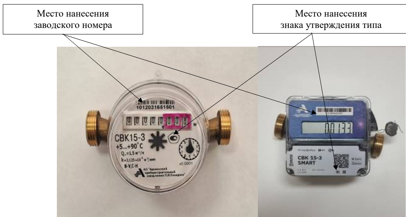
Рисунок 1 – Общий вид счетчиков с указанием места заводского номера и места нанесения знака утверждения типа
