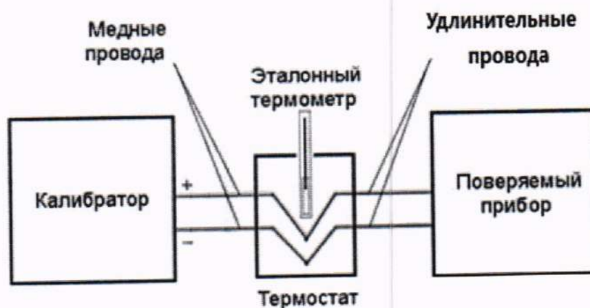
Рисунок 1 – Схема подключения
