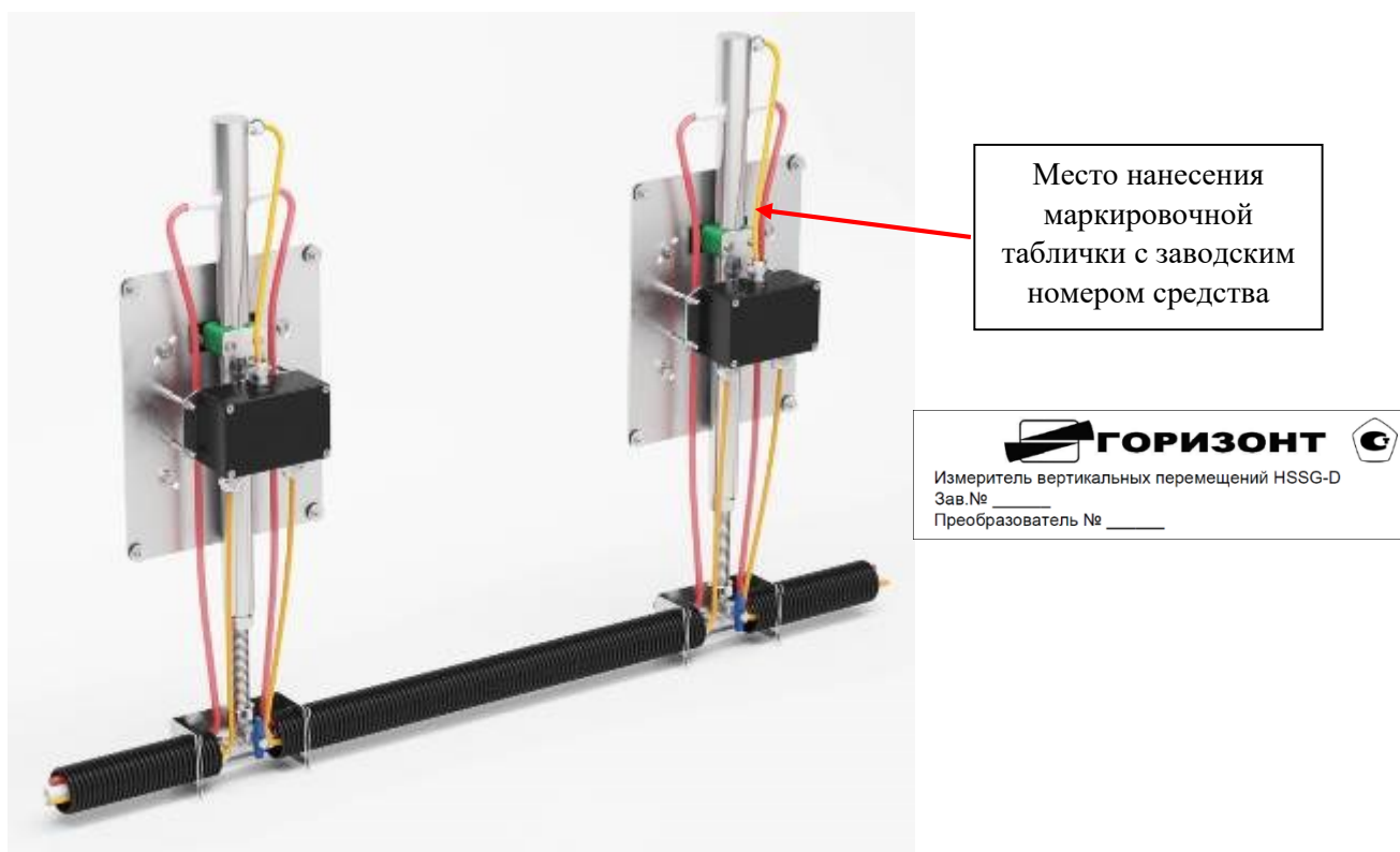
Рисунок 1 – Пример общего вида измерителя вертикальных перемещений HSSG-D
