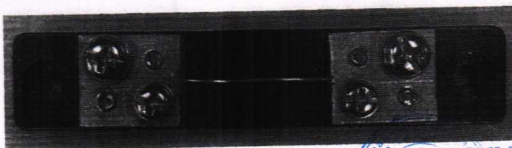
Рисунок 1.13 – Общий вид шунта, поставляемого в комплекте для модификаций Ц9256 с номинальным значением входного сигнала свыше 2 А до 10 А включительно
