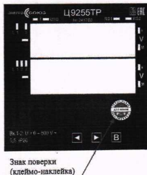
Рисунок 2.8 – Схема с указанием места для нанесения знака поверки на преобразователи Ц9254ТР, Ц9255ТР с двухстрочной многоцветной индикацией
