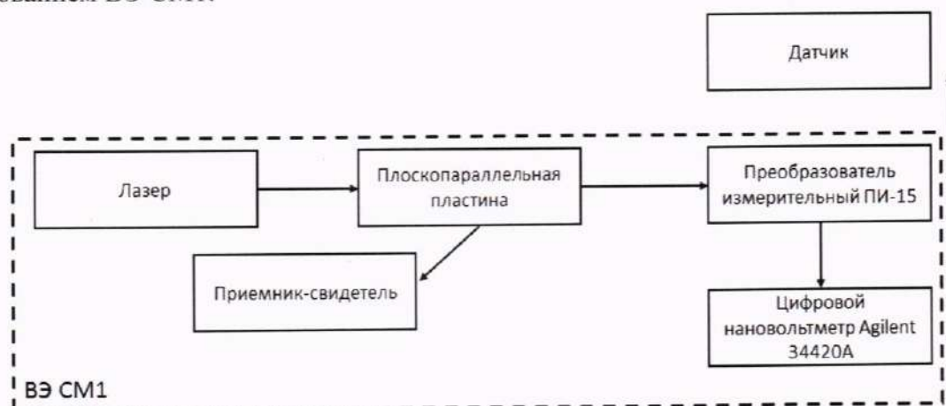
Рисунок 1 – Блок-схема подключения приборов для измерений с помощью ВЭ СМ1
