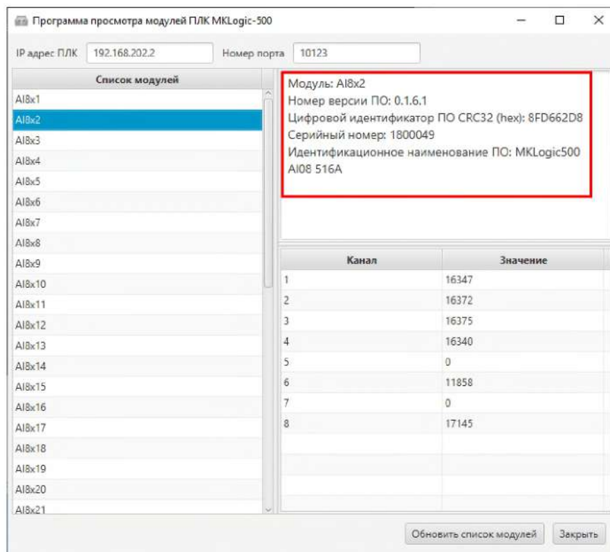
Рисунок 2 – Окно данных модулей ввода/вывода ПО «Программа просмотра модулей ПЛК MKLogic-500»
