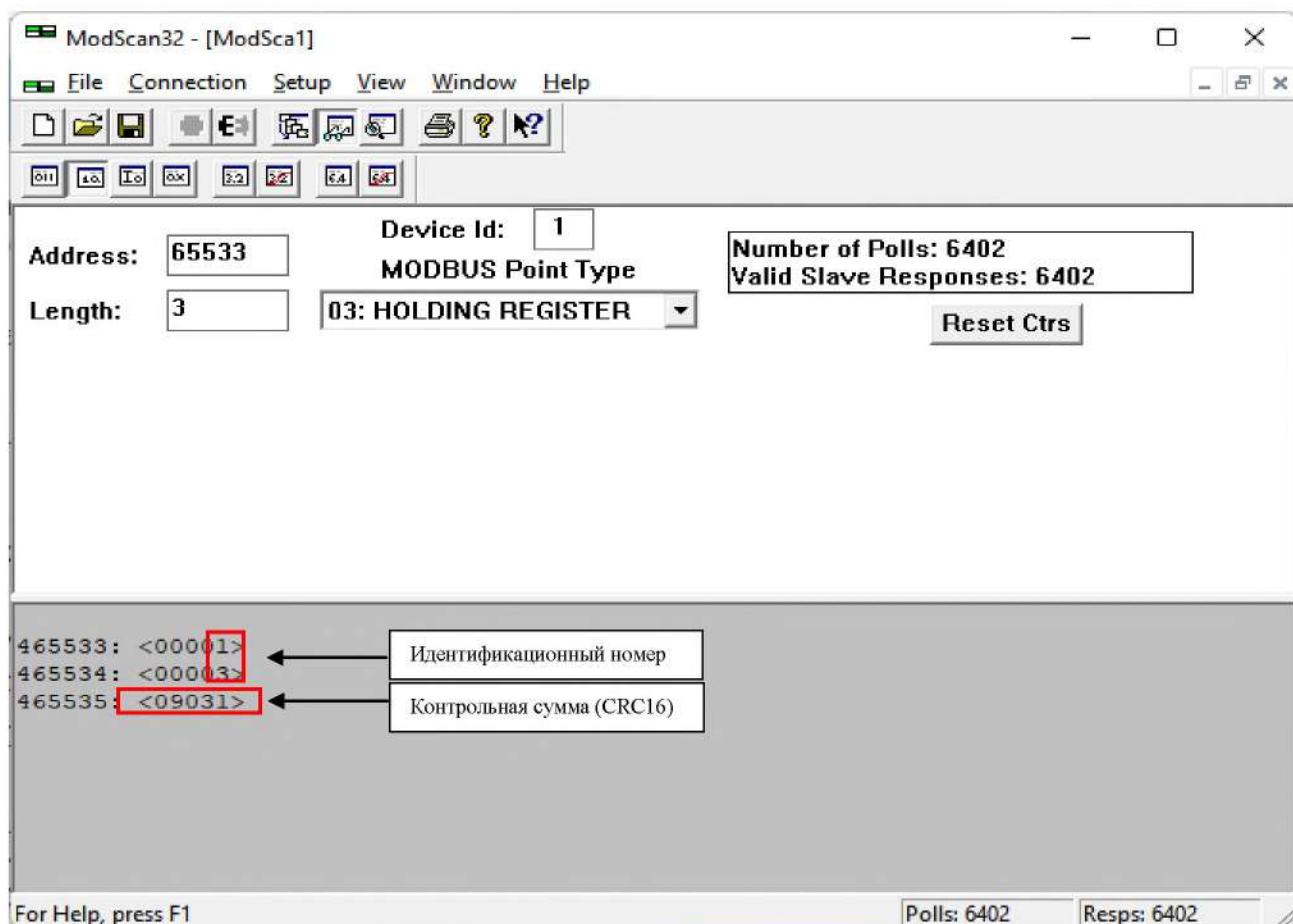
Рисунок 6 – Окно отображения идентификационного номера и контрольной суммы
