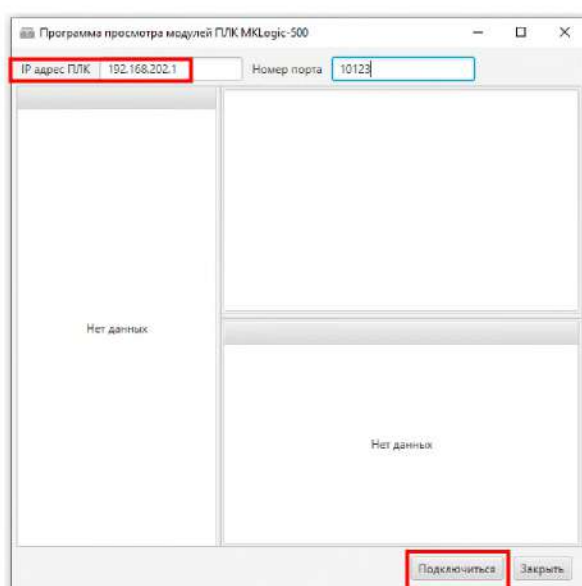
Рисунок 1 – Окно подключения ПО «Программа просмотра модулей ПЛК MKLogic-500»
