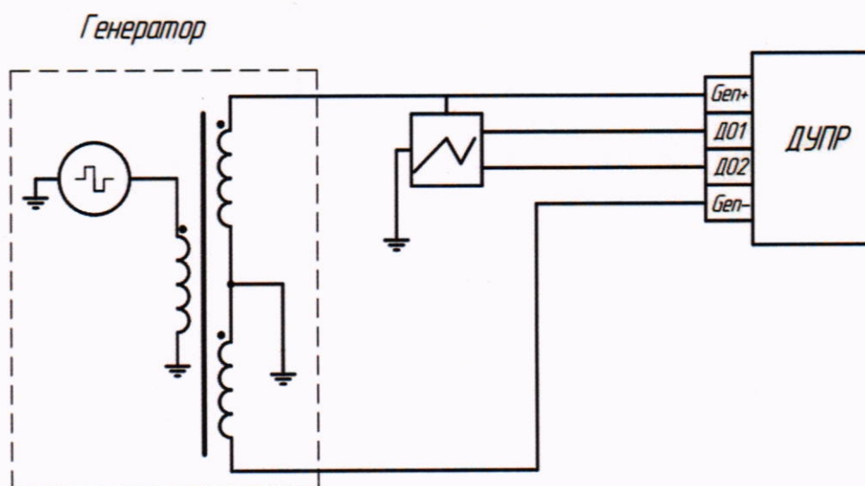
Рисунок 2 – Схема подключения
