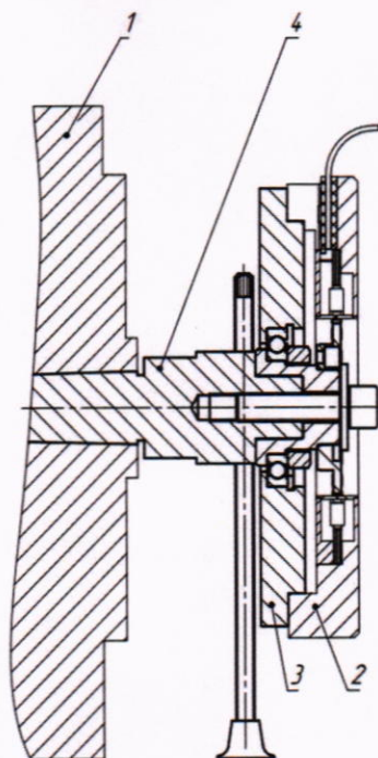
1 - головка делительная оптическая ОДГЭ-5; 2 - испытываемый датчик; 3 - корпус; 4 - хвостовик.
