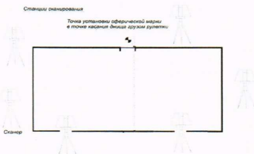
Рисунок А.3 - Схема сканирования внешней поверхности резервуара
