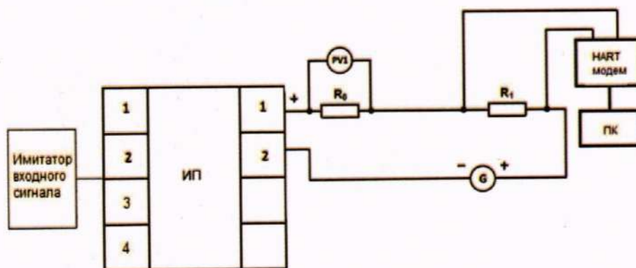
Рисунок Б.1 – Схема поверки преобразователя с прямым измерением токового сигнала и подключением HART-модема
