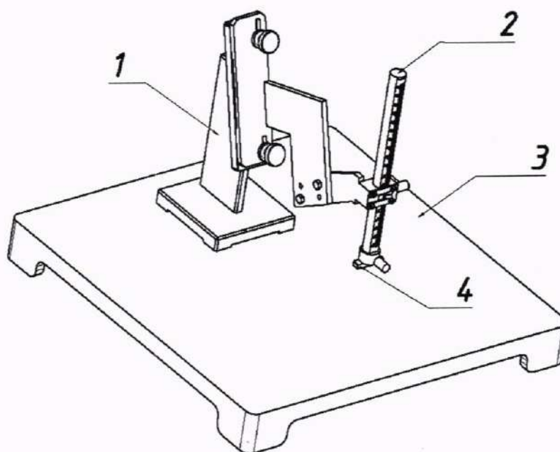
1 – штатив; 2 – линейка; 3 – рабочая поверхность; 4 – измерительная поверхность Рисунок 1 – Установка приспособления
