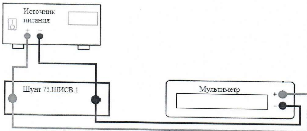
Рисунок 4 – Структурная схема соединения приборов
