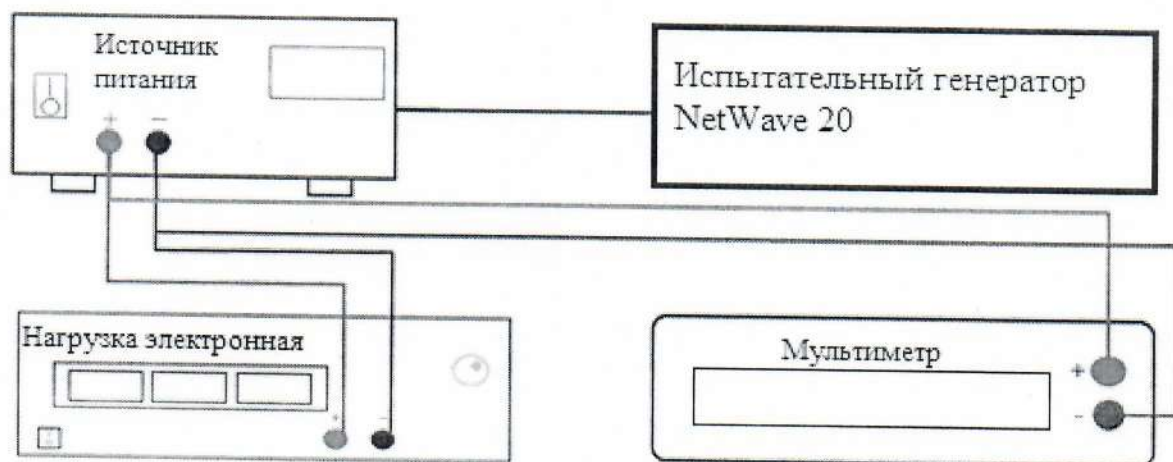
Рисунок 2 – Структурная схема соединения приборов
