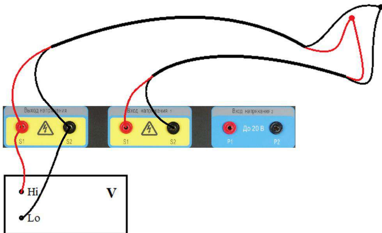
Рисунок 1 – Схема измерений среднеквадратических значений напряжения переменного тока синусоидальной формы
