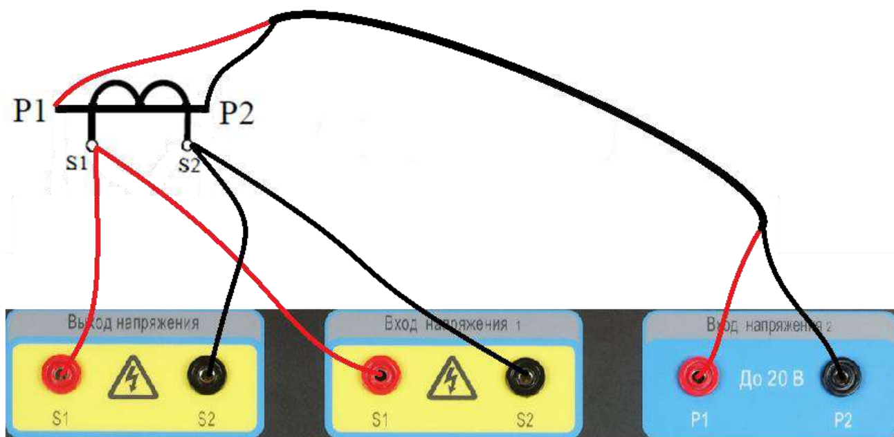
Рисунок 4 – Схема измерений коэффициента трансформации и угла фазового сдвига трансформатора тока
