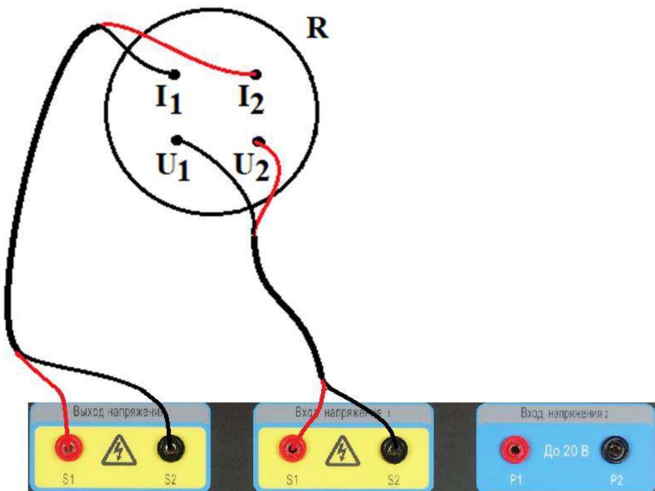
Рисунок 3 – Схема измерений электрического сопротивления постоянному току
