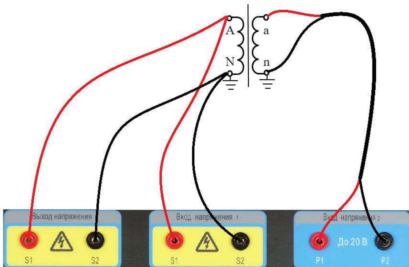
Рисунок 5 – Схема измерений коэффициента трансформации трансформатора напряжения
