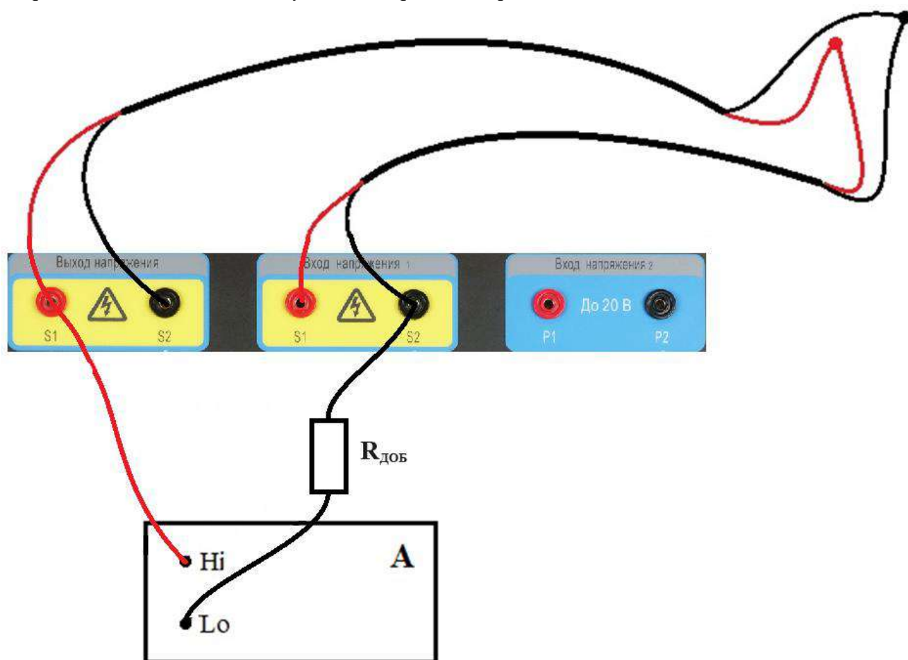
Рисунок 2 – Схема измерений среднеквадратических значений силы переменного тока синусоидальной формы
