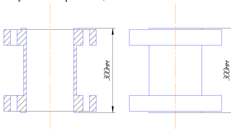
Рисунок А.2 Проставка, номинальной высотой 300 мм
