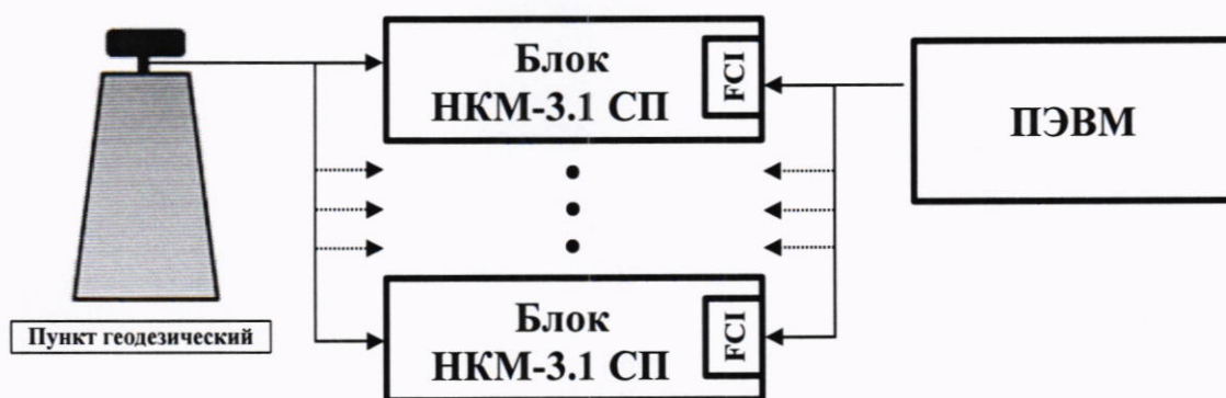
Рисунок 7 – Схема проведения измерений при определении абсолютной погрешности (при доверительной вероятности 0,95) определения координат местоположения по каждой координатной оси при работе по сигналам ГЛОНАСС (L1, код СТ) и GPS (L1, код C/A) при геометрическом факторе PDOP не более 3
