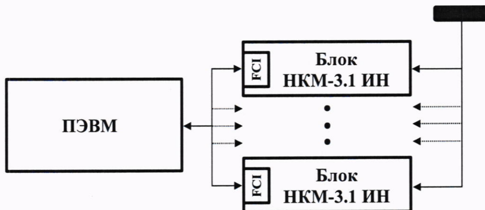
Рисунок 4 – Схема проведения опробования блоков НКМ-3.1 ИН (метод 2)
