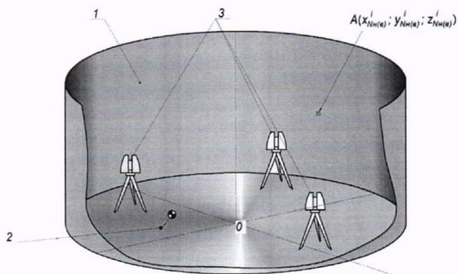
1 – внутренняя полость резервуара; 2 – точка установки марки в точке касания дна груза рулетки; 3 – точки стояния станций съемки
