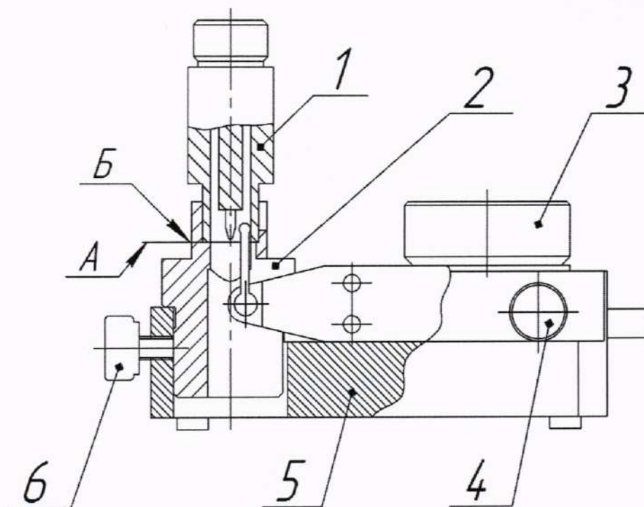
Рисунок 1 – Измеритель несоосности
