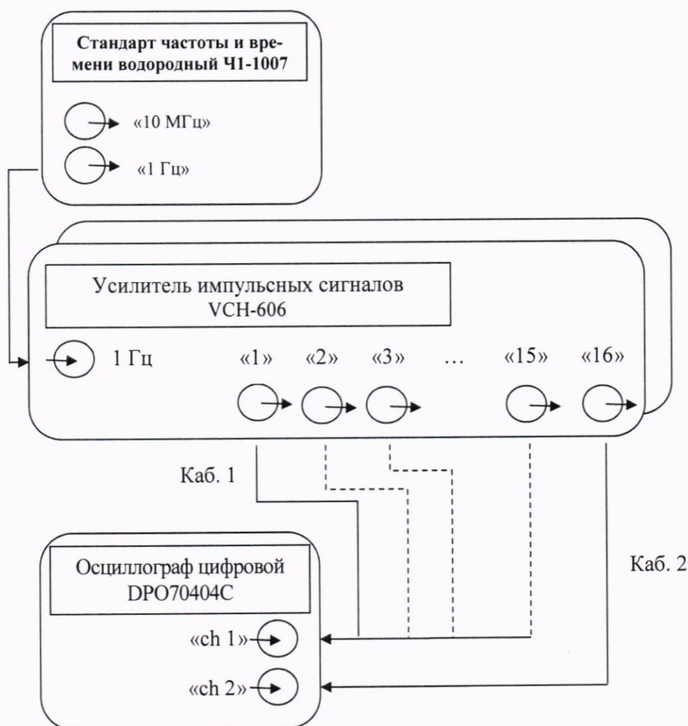
Рисунок 2 – схема определения значений задержек сигналов на выходных разъемах усилителей импульсных сигналов VCH-606
