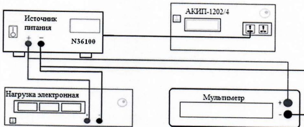
Рисунок 2 – Структурная схема соединения приборов
